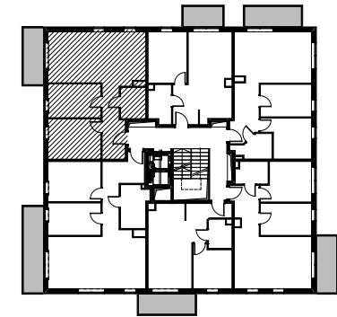
Rzut kondygnacji z lokalizacją mieszkania
