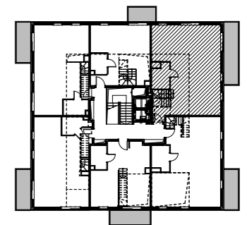
Rzut kondygnacji z lokalizacją mieszkania - IV piętro
