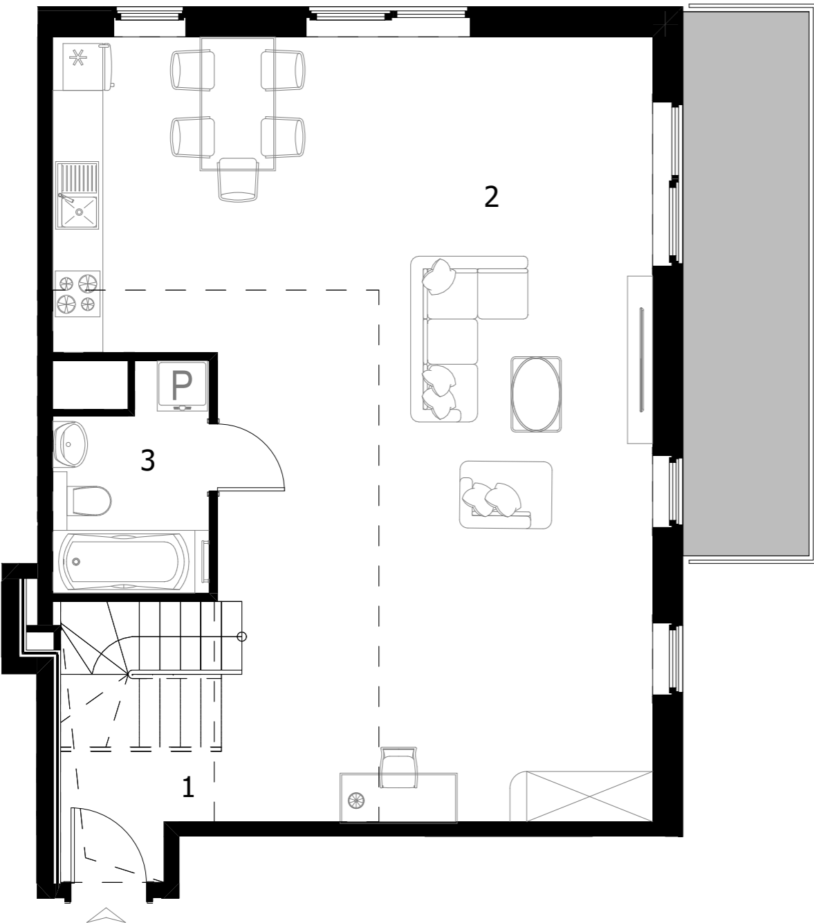
Rzut lokalu mieszkalnego - IV piętro
