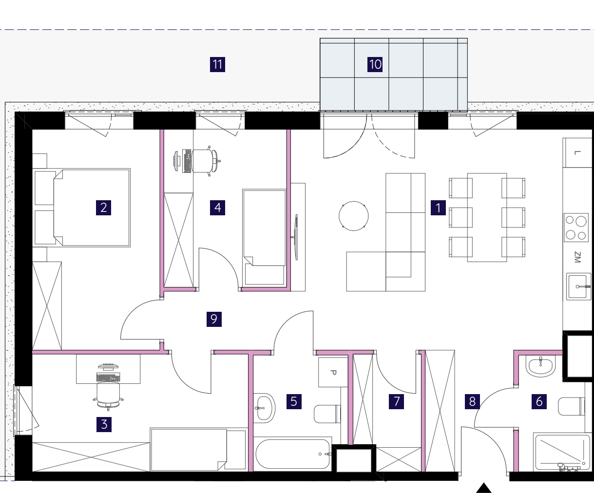
Rzut z pokazaniem ogródka
