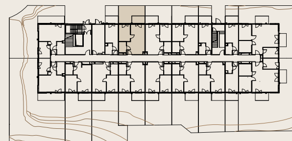
Rzut kondygnacji - parter - budynek B
