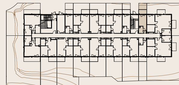
Rzut kondygnacji - parter - budynek B
