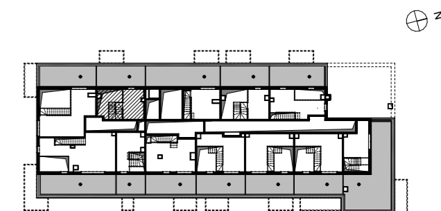
Rzut kondygnacji z lokalizacją mieszkania - IV piętro
